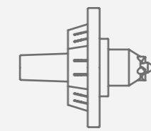
Stirnmittnehmer / Morsekegel Adaption zur Spitzenspannung
